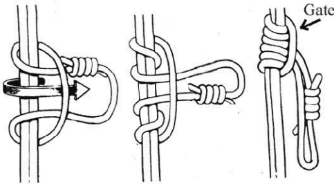
Prusik
